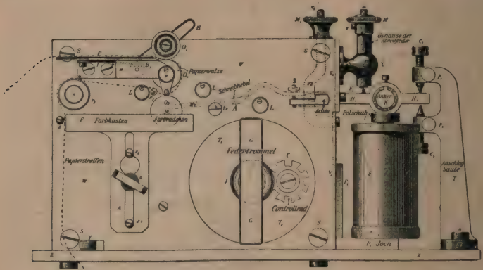
Morseapparat. Aus Hamacher, Telegraphie und Telephonie.
